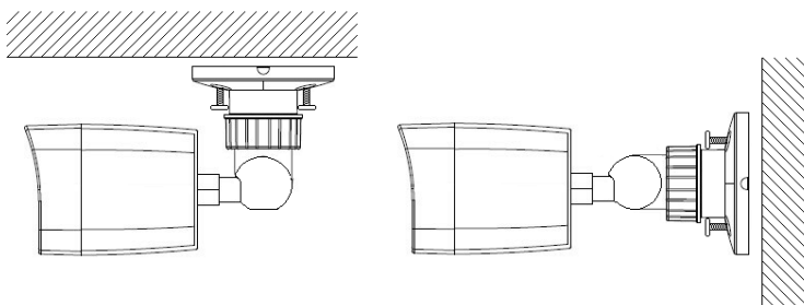
Figura 2.2 Parafuse a câmera ao teto ou a parede
