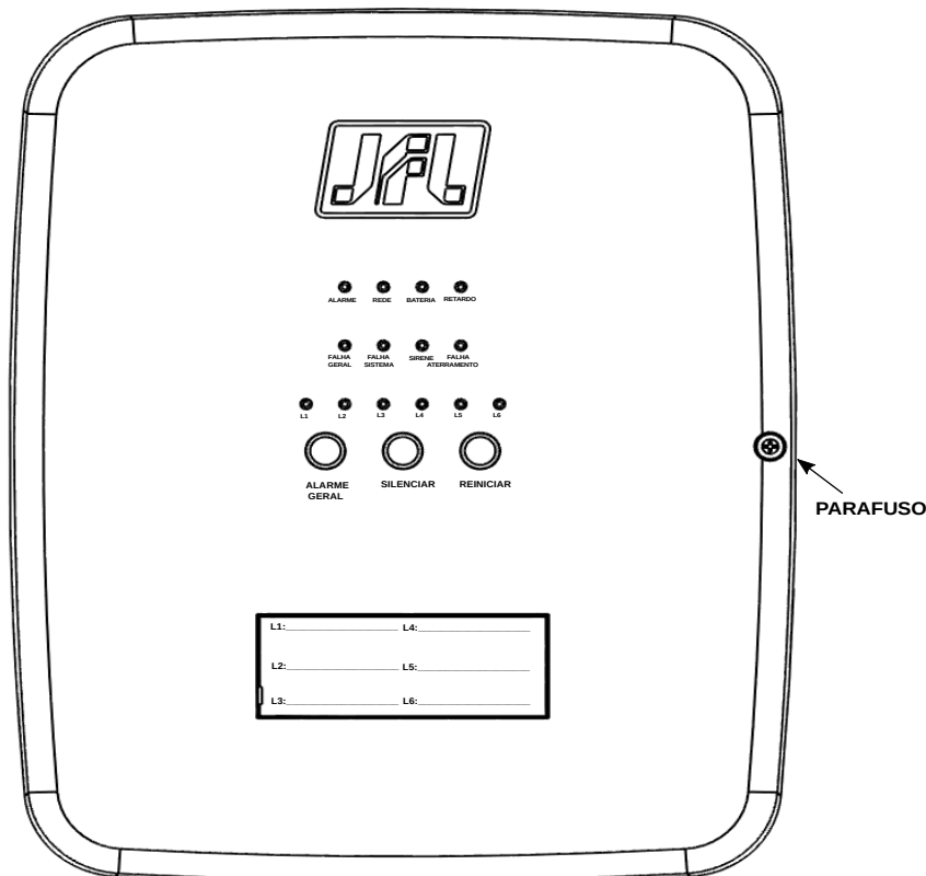
Figura 2: Vista frontal
